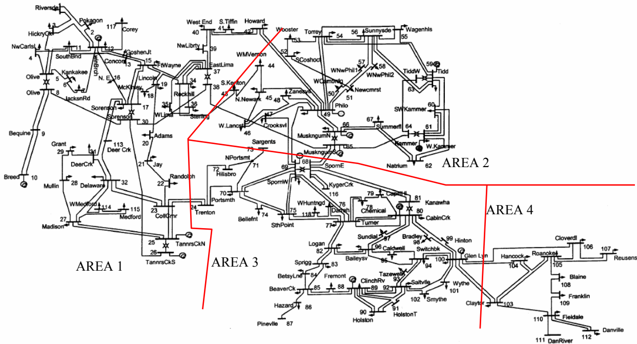
Fig. 1. The 118-bus test system.
